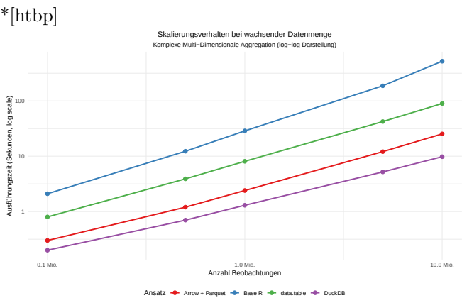
Abbildung 3: Skalierungsverhalten verschiedener Ansätze (Szenario B: Komplexe Aggregation)
