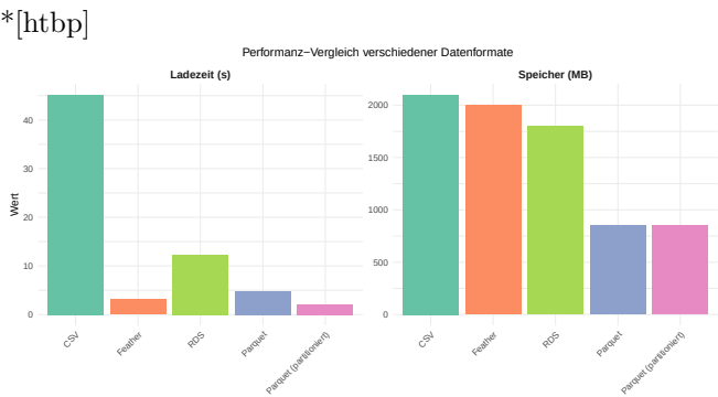
Abbildung 2: Ladezeiten verschiedener Datenformate (BTP-Datensatz, 5 Mio. Zeilen, 50 Variablen)
