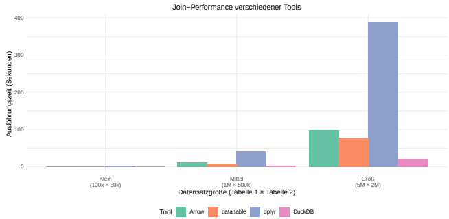
Abbildung 5.3: Join-Performance bei verschiedenen Datensatzgrößen (Inner Join zweier Tabellen)
