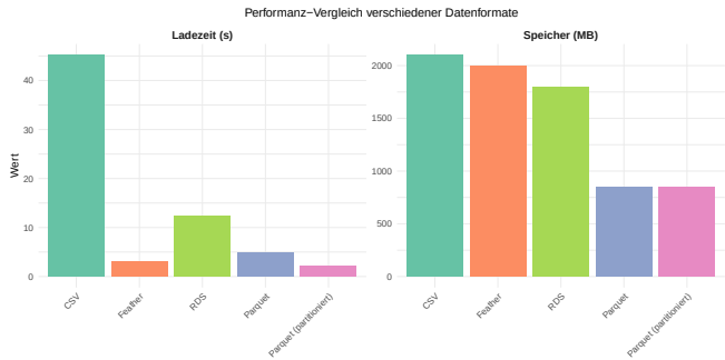
Abbildung 5.1: Ladezeiten verschiedener Datenformate (BTP-Datensatz, 5 Mio. Zeilen, 50 Variablen)
