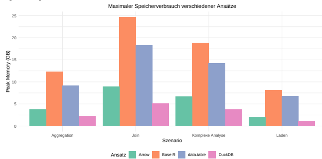
Abbildung 5.4: Peak Memory Usage verschiedener Ansätze (5 Mio. Zeilen)
