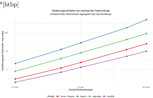
Abbildung 5.2: Skalierungsverhalten verschiedener Ansätze (Szenario B: Komplexe Aggregation)
