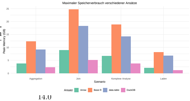
Abbildung 5: Peak Memory Usage verschiedener Ansätze (5 Mio. Zeilen)
