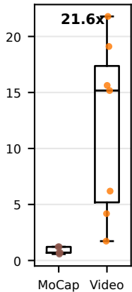
M1 torso-length CV [%]
