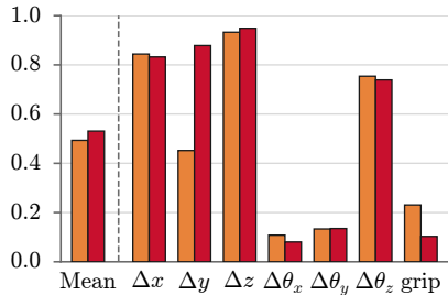
MLP R^2 per action dim.
