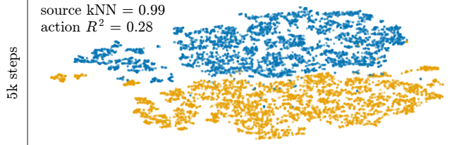
DINOv3 encoder
