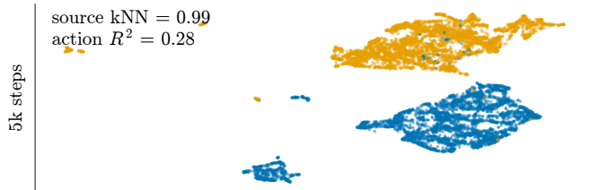
DINOv3 encoder
