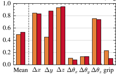
MLP R^2 per action dim.
