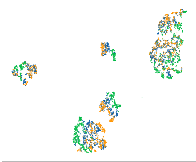
1k steps
