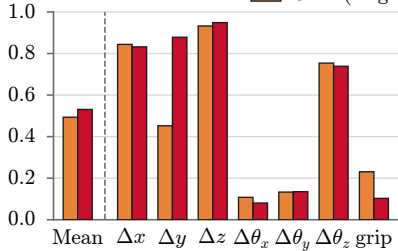
MLP R^2 per action dim.
