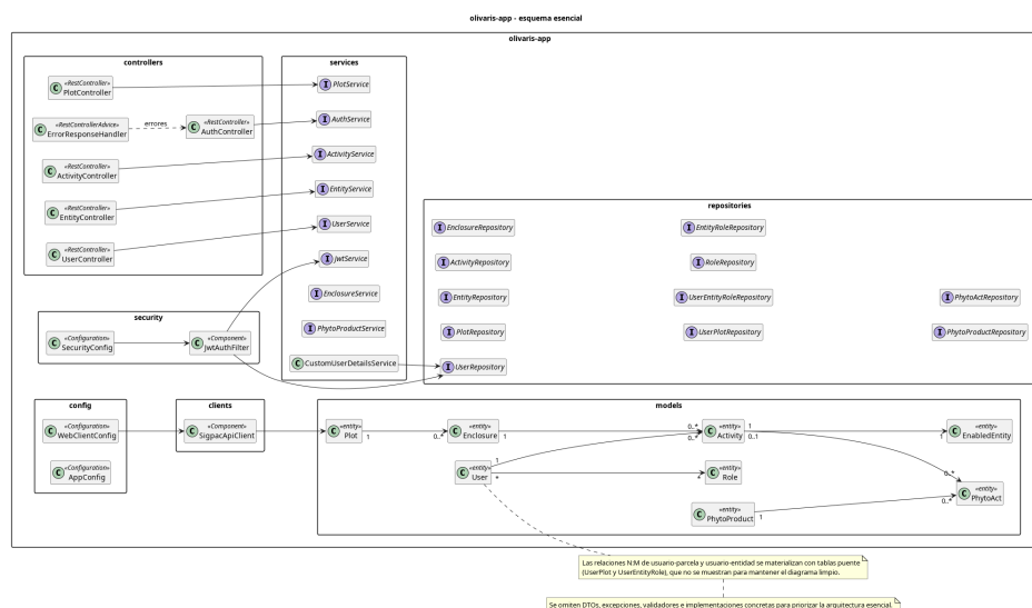
Figura 6.3: Diagrama de clases
