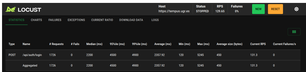
Figura 8.6: Estadísticas para 1000 usuarios en el login desde on premise
