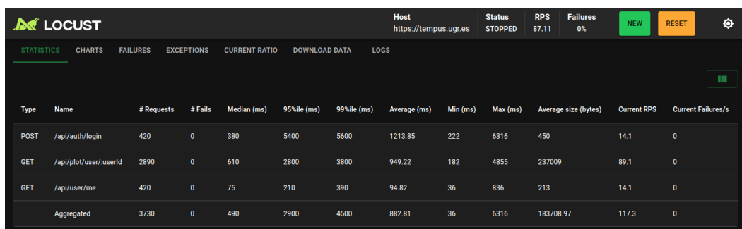
Figura 8.7: Estadísticas para 1000 usuarios en la obtención de parcelas
