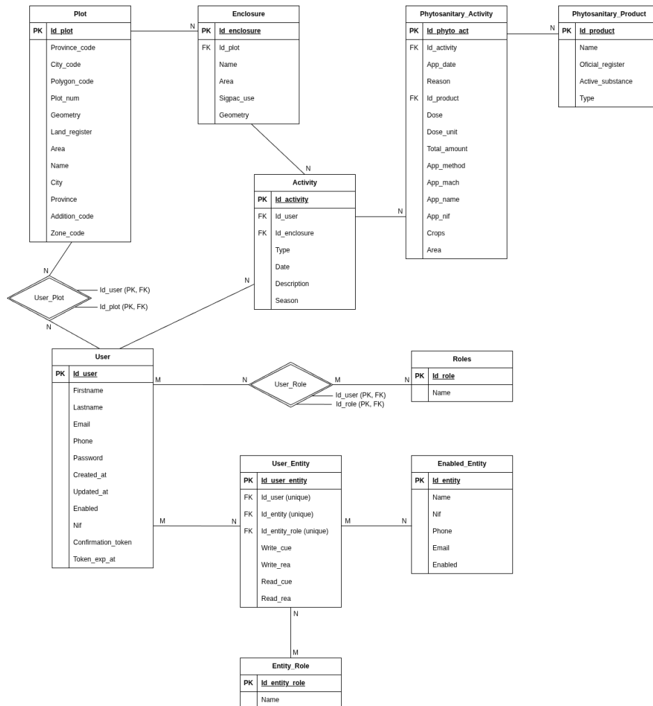
Figura 6.2: Diagrama E/R de la base de datos
