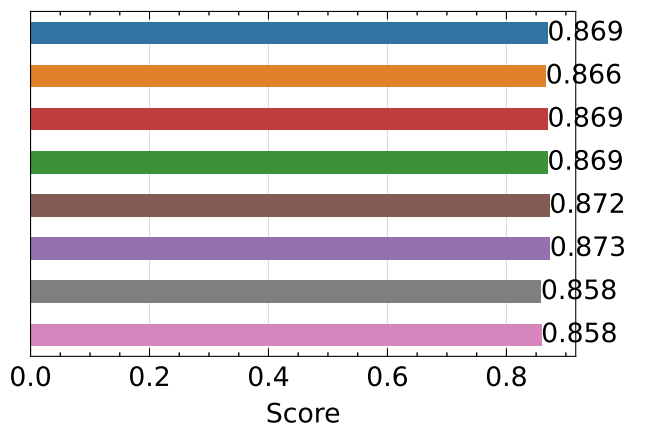
SSIM ↑
