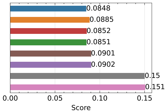
LPIPS ↓
