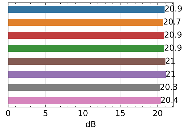
PSNR ↑
