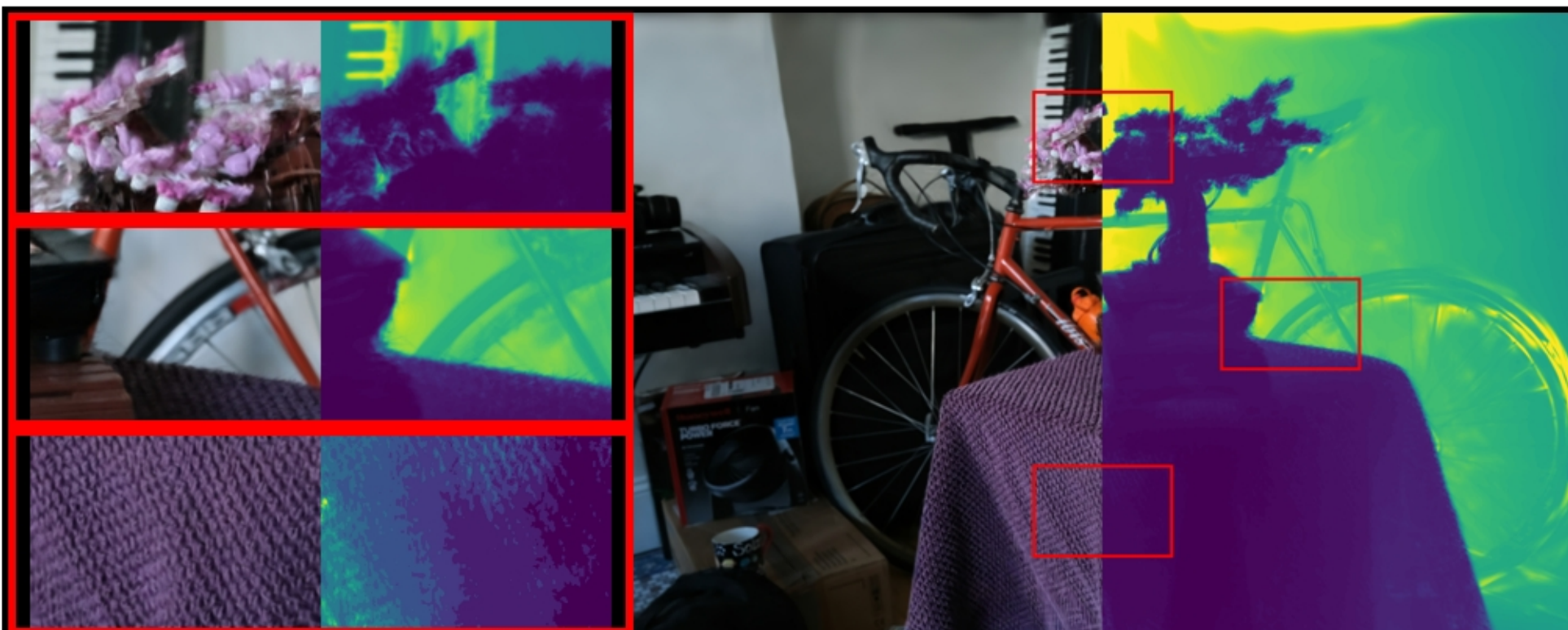
bonsai: VGGT | depth_lambda=1.0 PSNR: 17.64 | LPIPS: 0.3894 | SSIM: 0.5626
