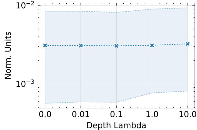
SSIM ↑
