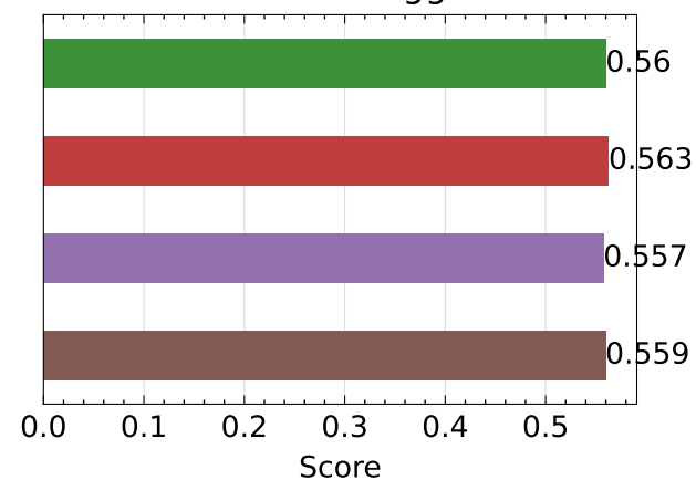
SSIM ↑ - vgg
