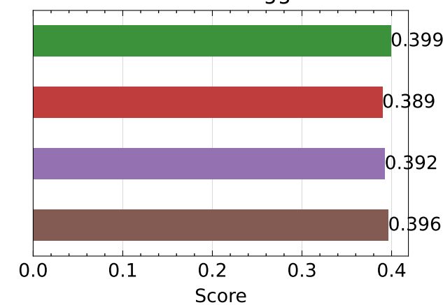
LPIPS ↓ - vgg
