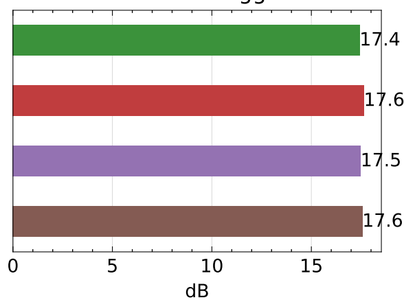
PSNR ↑ - vgg
