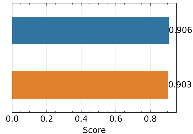
RRE ↓ - vgg
