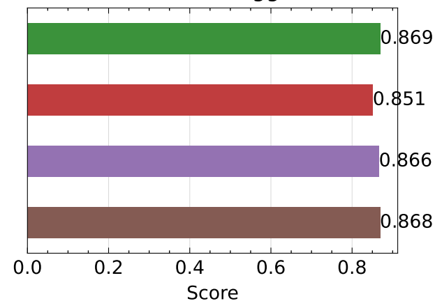
SSIM ↑ - vgg
