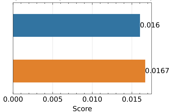
LPIPS ↓ - vgg
