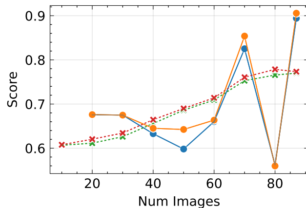
SSIM ↑
