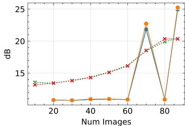
PSNR ↑
