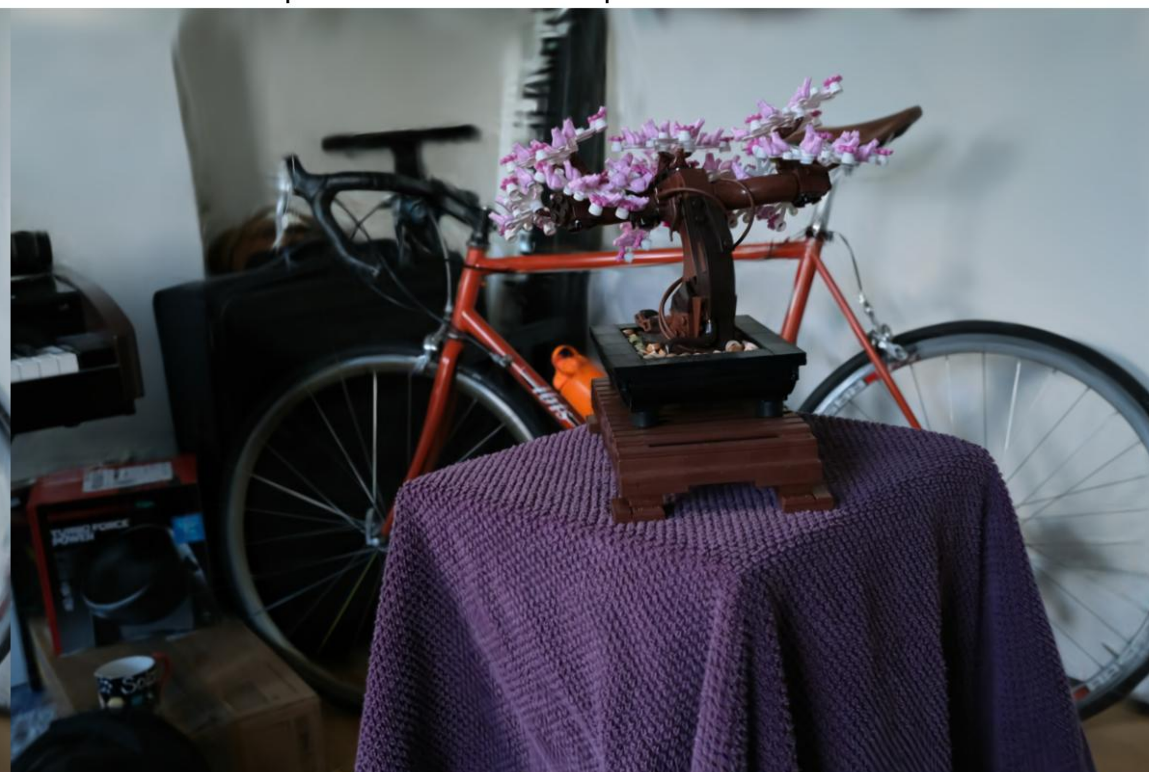
Config: VGGT | voxels | num_points=100000 PSNR: 27.70 | LPIPS: 0.1406 | SSIM: 0.9167
