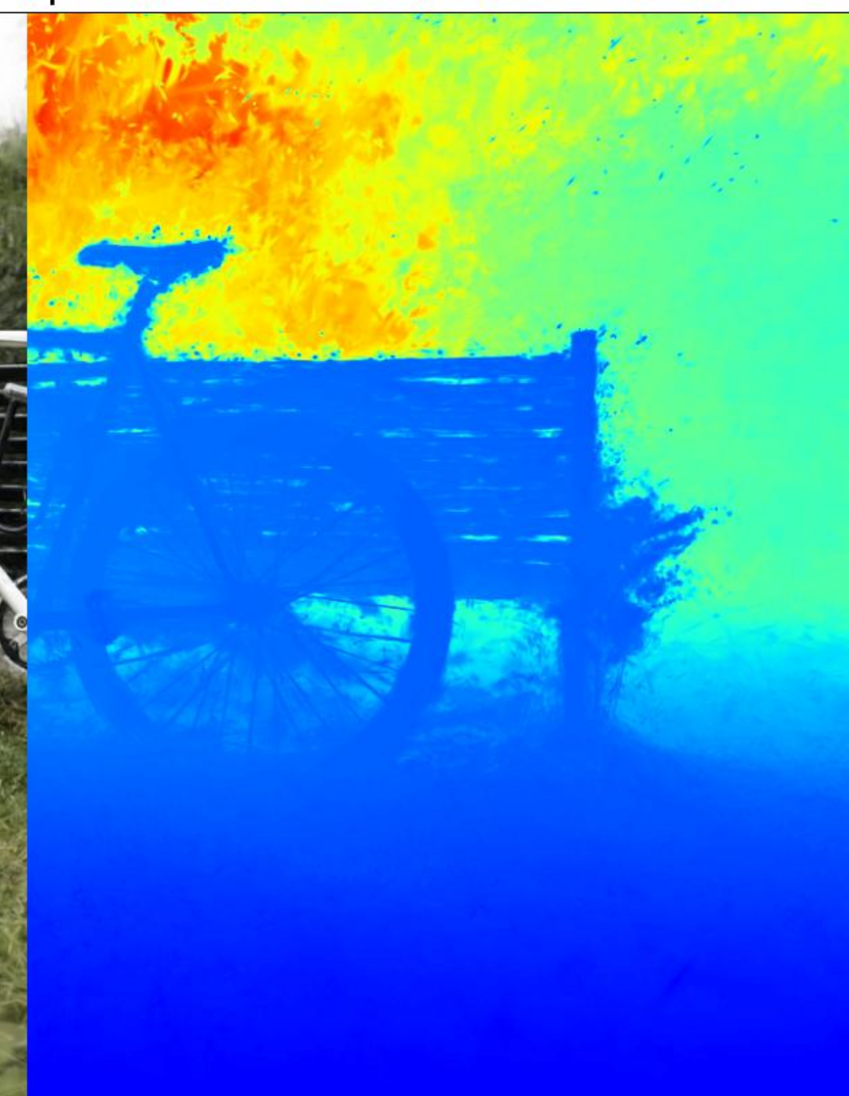
Config: VGGT | | points | depth_lambda=1.0 PSNR: 15.77 | LPIPS: 0.4046 | SSIM: 0.2093
