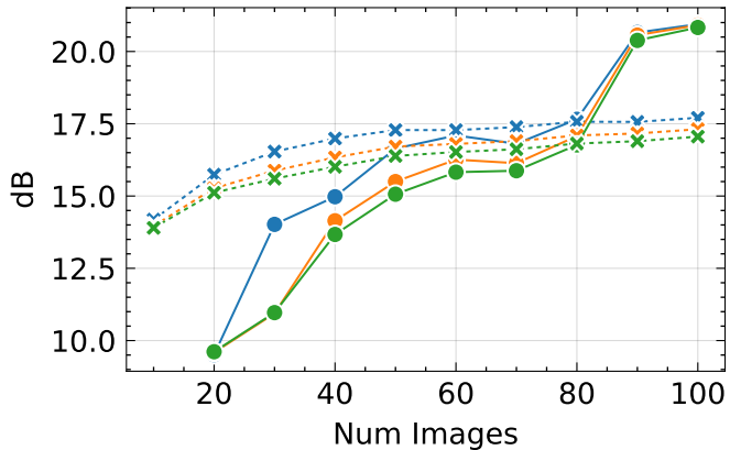
PSNR \uparrow
