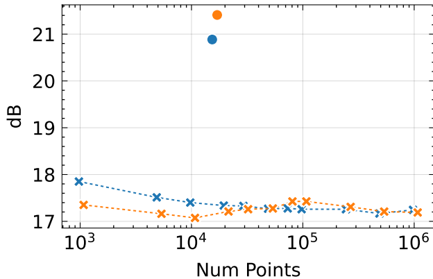
PSNR \uparrow
