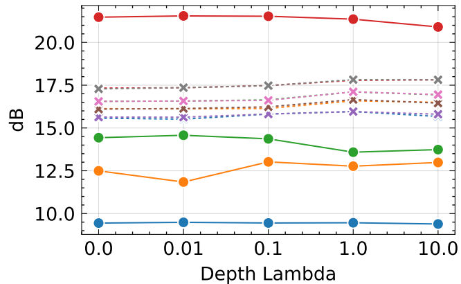
PSNR \uparrow
