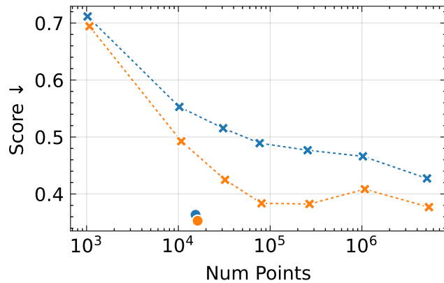
LPIPS
