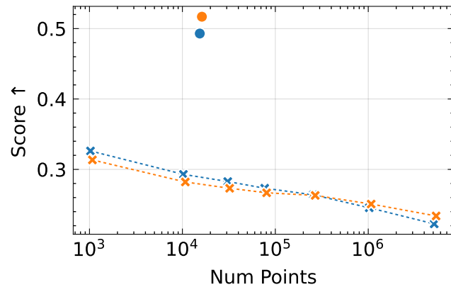
SSIM
