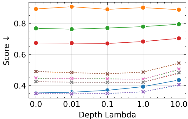
LPIPS
