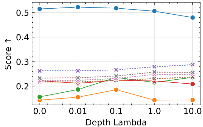
SSIM
