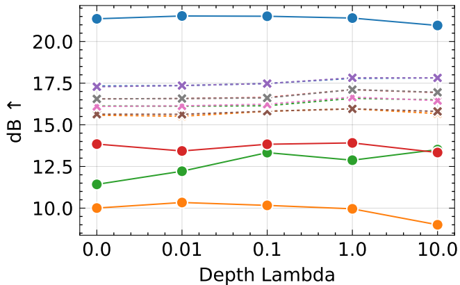
PSNR
