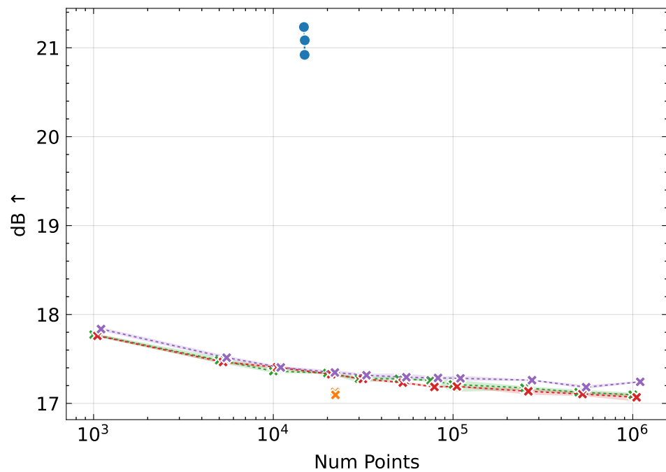
PSNR
