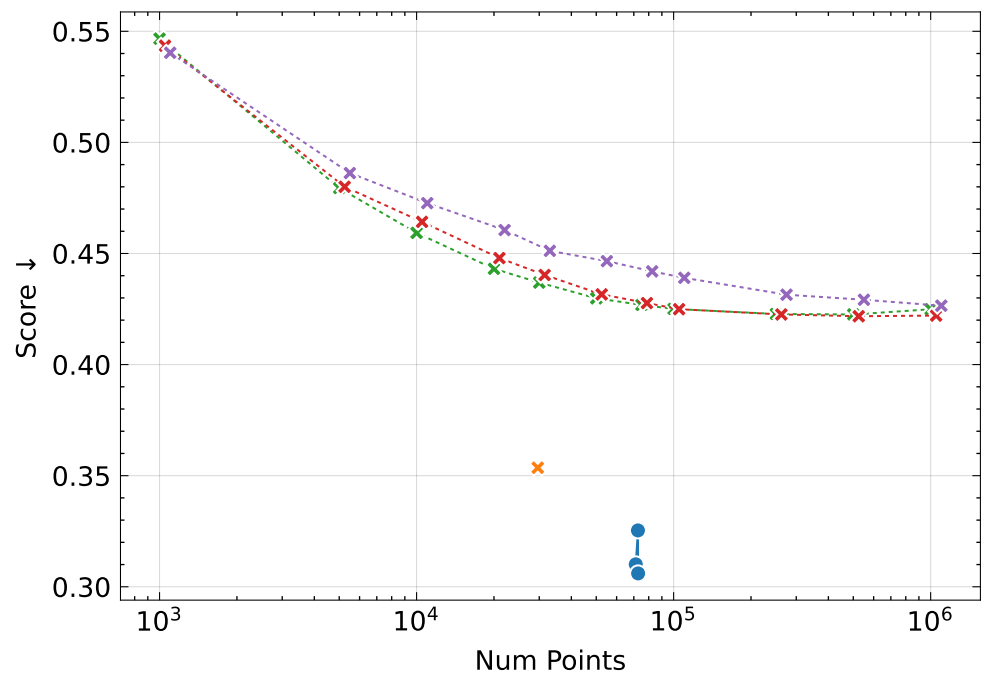
LPIPS
