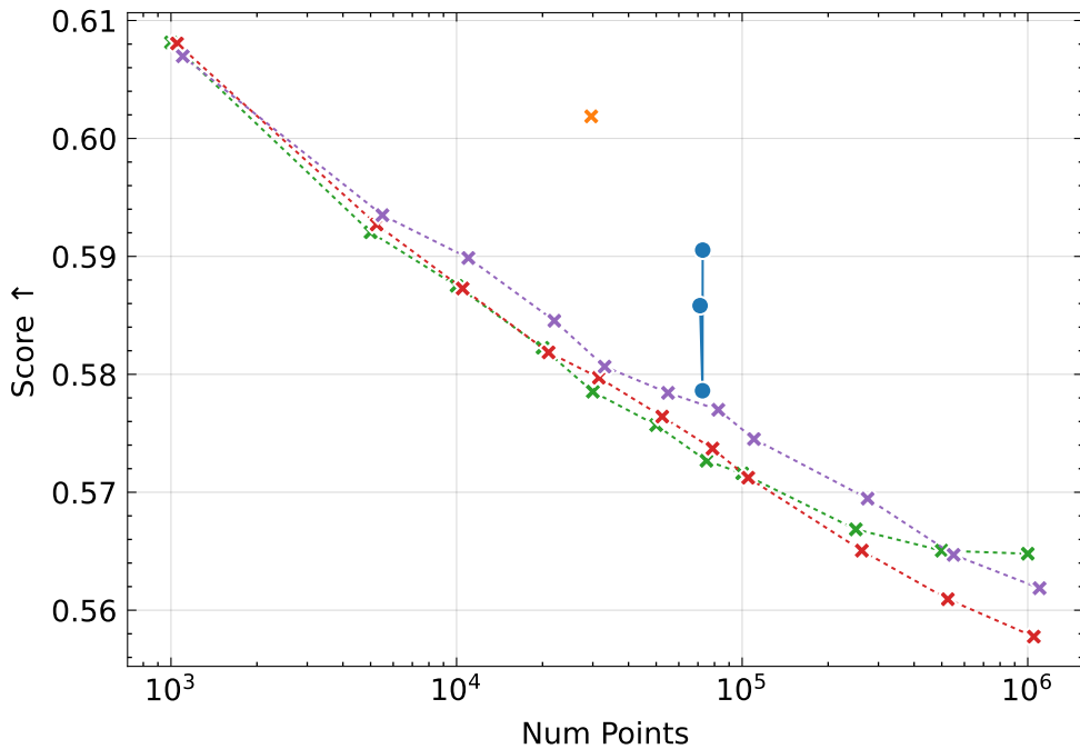
SSIM
