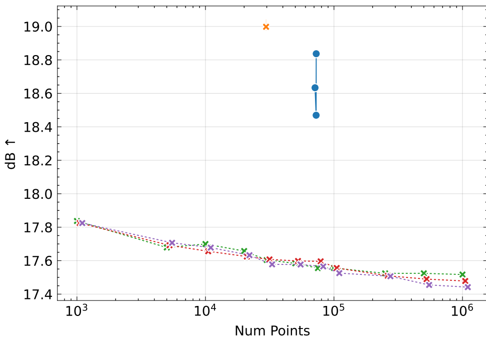
PSNR
