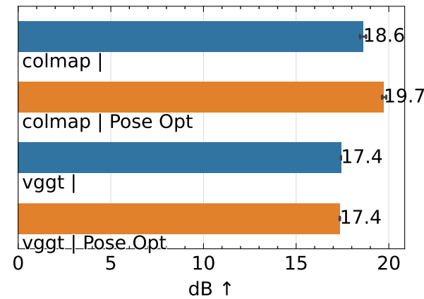
PSNR
