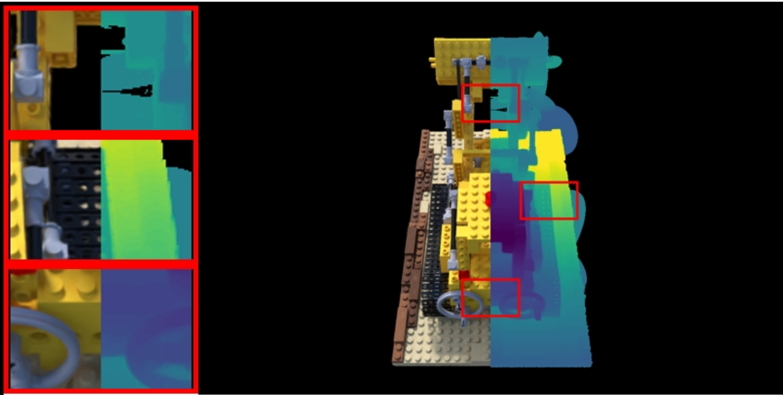
lego: VGGT | PSNR: 21.97 | LPIPS: 0.0697 | SSIM: 0.8123
