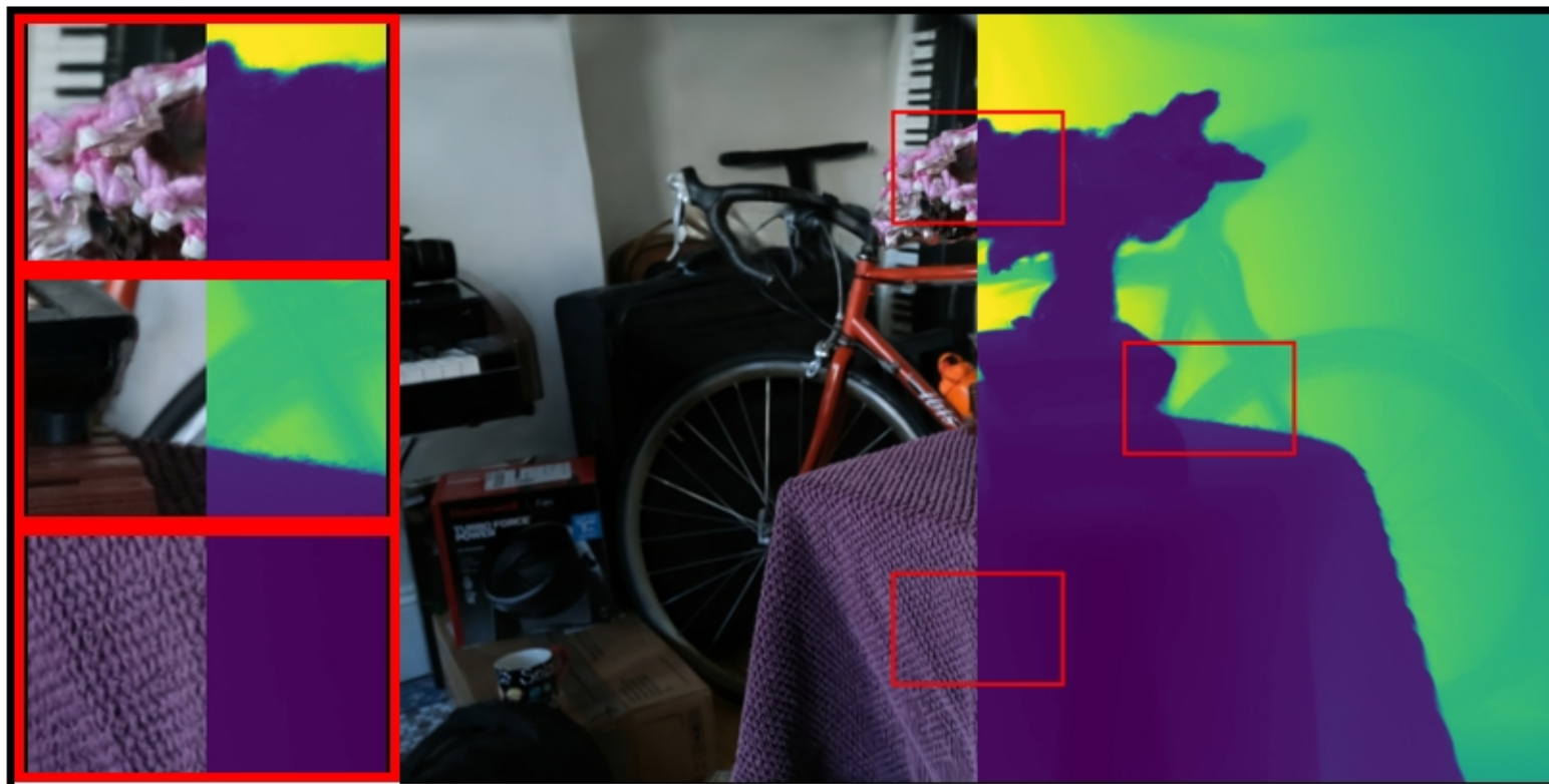
bonsai: VGGT | sigmoid PSNR: 17.48 | LPIPS: 0.3911 | SSIM: 0.5575
