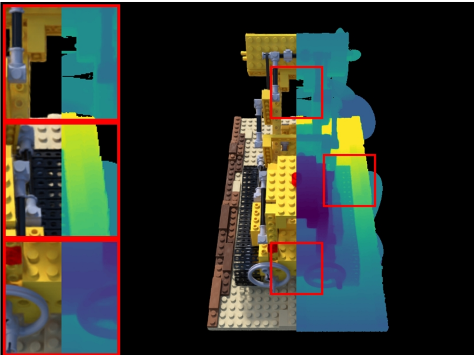
lego: VGGT | PSNR: 21.97 | LPIPS: 0.0697 | SSIM: 0.8123
