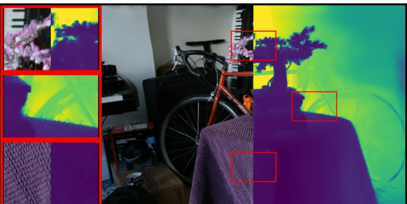
bonsai: VGGT | PSNR: 17.42 | LPIPS: 0.3988 | SSIM: 0.5598
