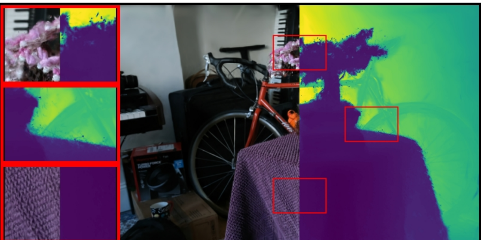
bonsai: VGGT | points PSNR: 17.56 | LPIPS: 0.3961 | SSIM: 0.5594
