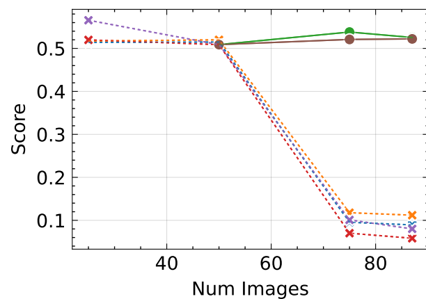
LPIPS ↓
