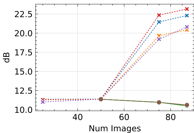
PSNR ↑
