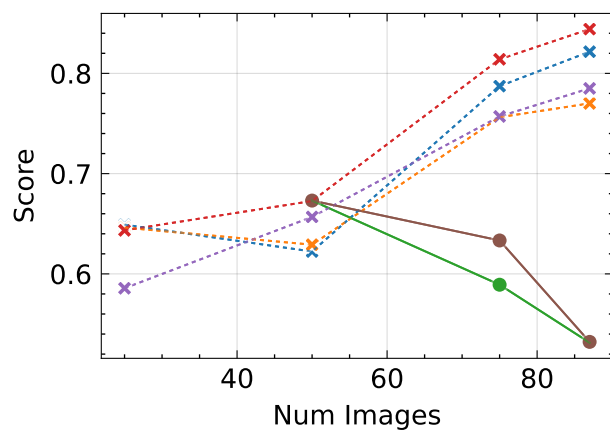
SSIM ↑
