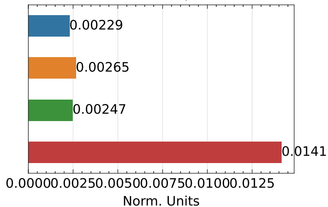
SSIM ↑
