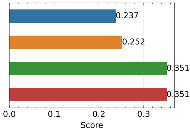
LPIPS ↓
