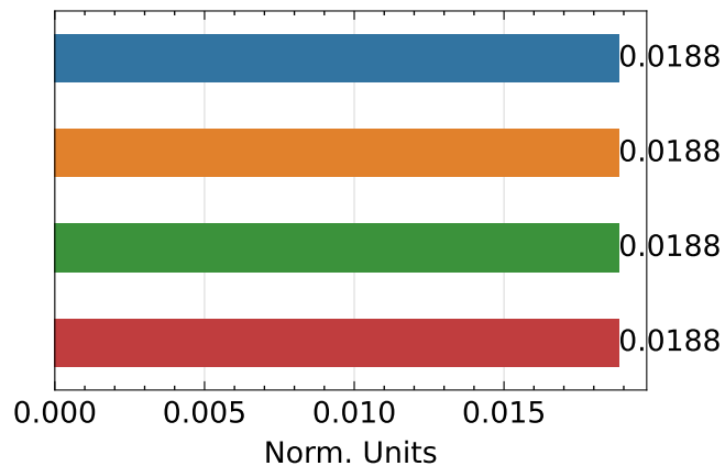
SSIM ↑
