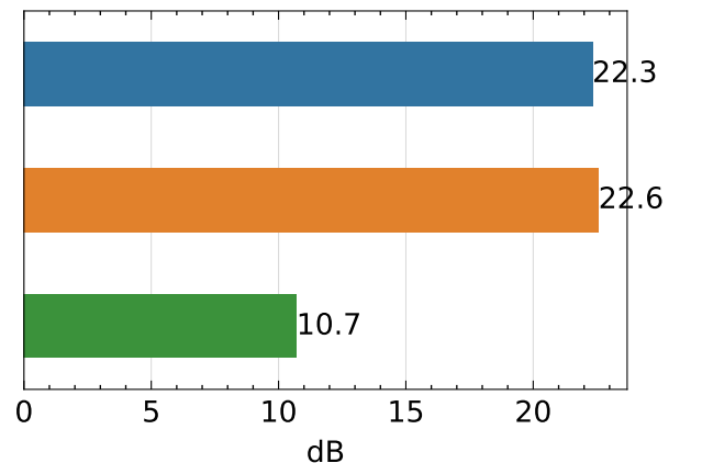
PSNR ↑
