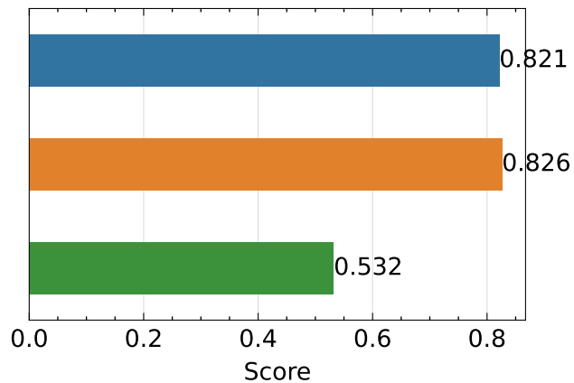
SSIM ↑
