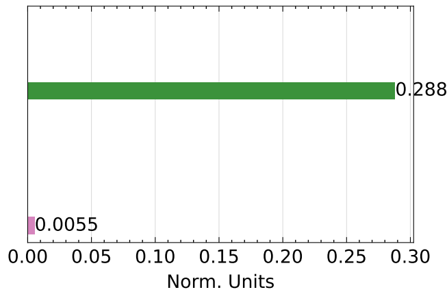
SSIM ↑
