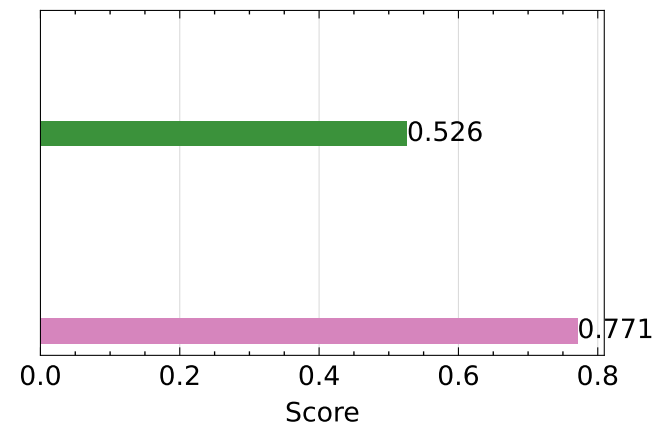
SSIM ↑
