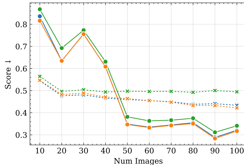
LPIPS
