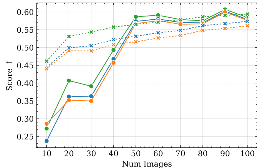
SSIM
