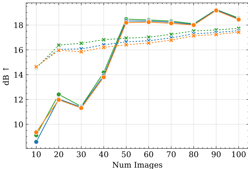
PSNR
