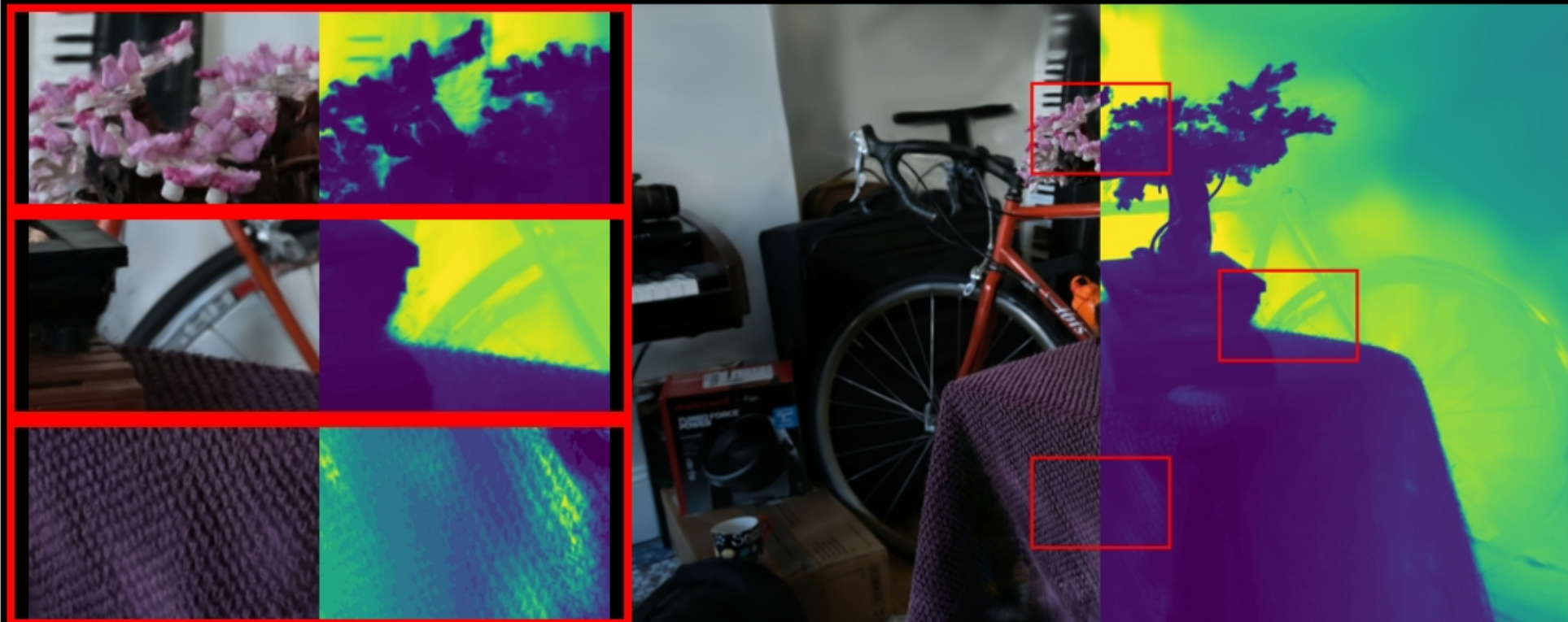
bonsai: VGGT | PSNR: 18.46 | LPIPS: 0.3355 | SSIM: 0.5824
