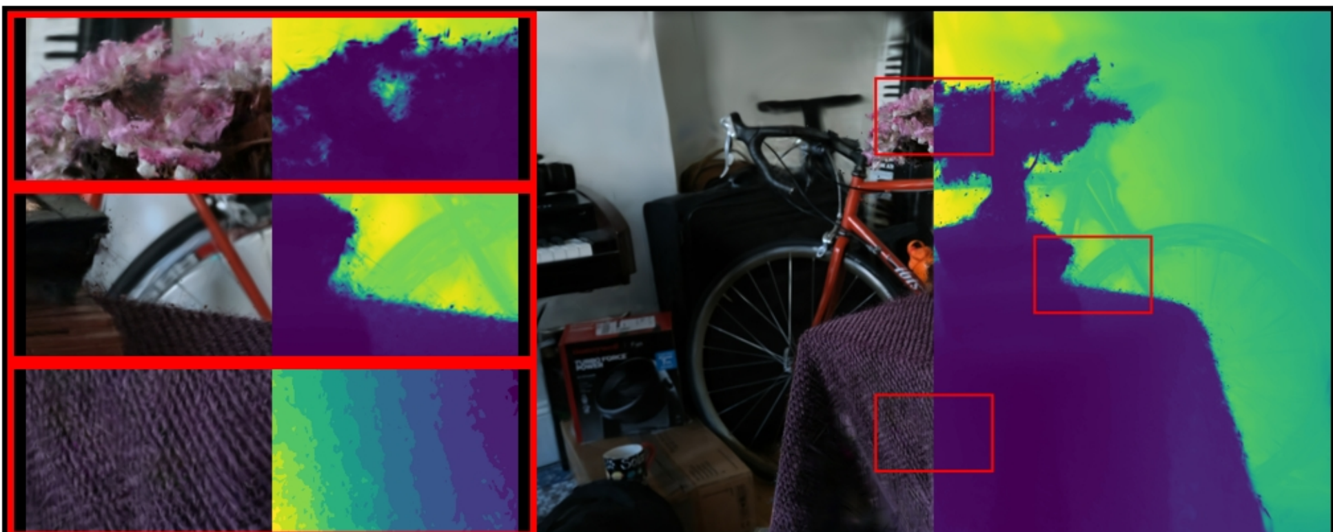
bonsai: VGGT | points PSNR: 18.56 | LPIPS: 0.3459 | SSIM: 0.5859
