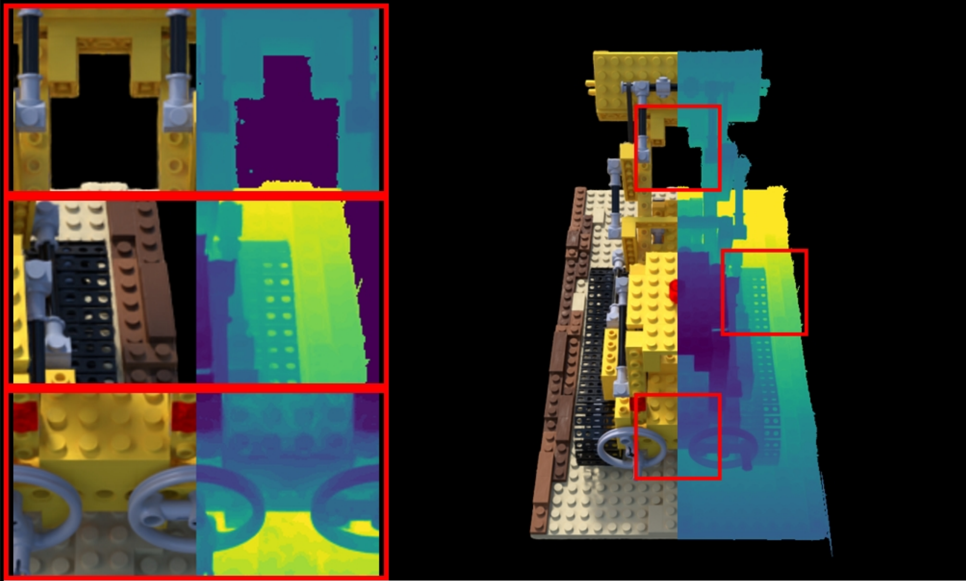
lego: VGGT | PSNR: 20.35 | LPIPS: 0.0759 | SSIM: 0.7735
