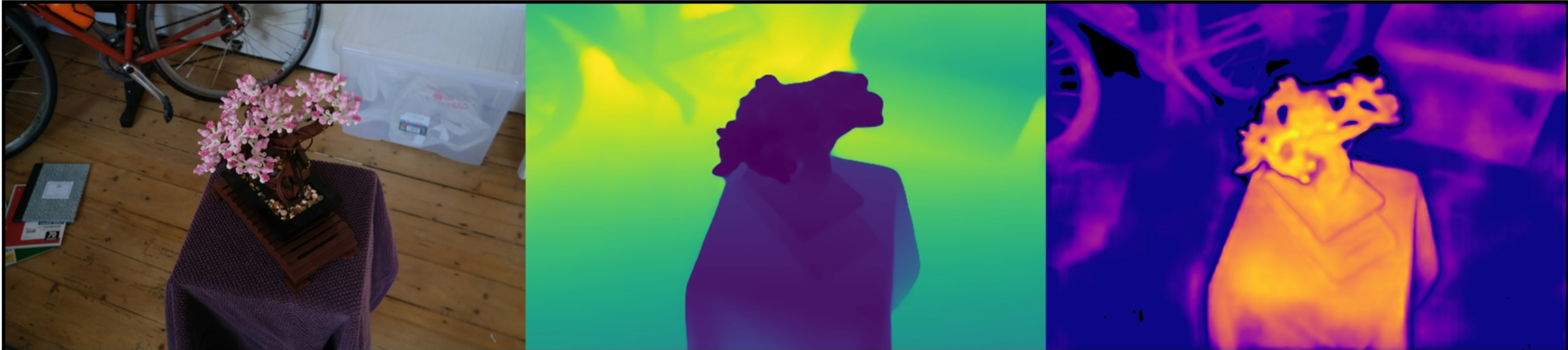
bonsai: VGGT Original | Depth (max=1.83) | Confidence (max=3.83)
