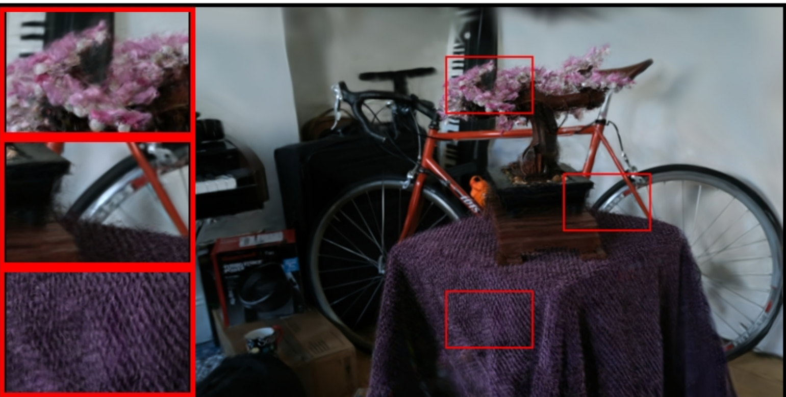
bonsai: VGGT | num_images=100 PSNR: 18.66 | LPIPS: 0.3740 | SSIM: 0.5956
