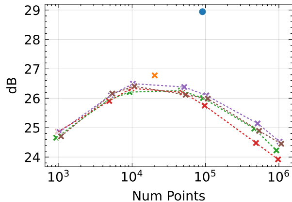
PSNR \uparrow
