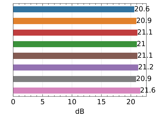
PSNR ↑ - counter
