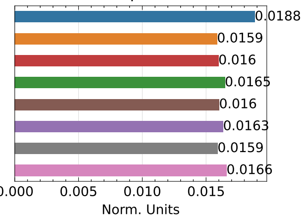
PSNR ↑ - bonsai
