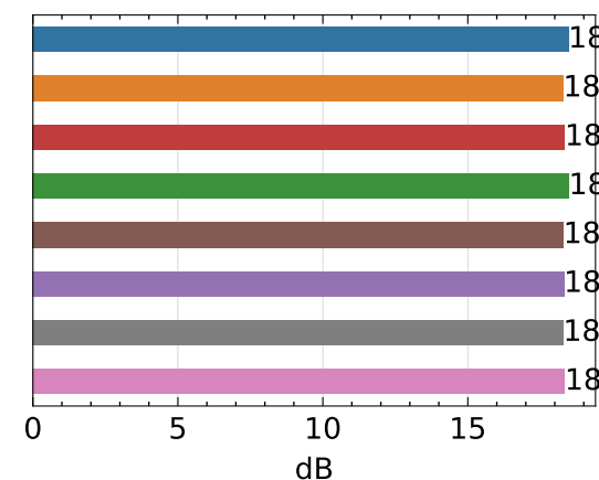
PSNR ↑ - bonsai
