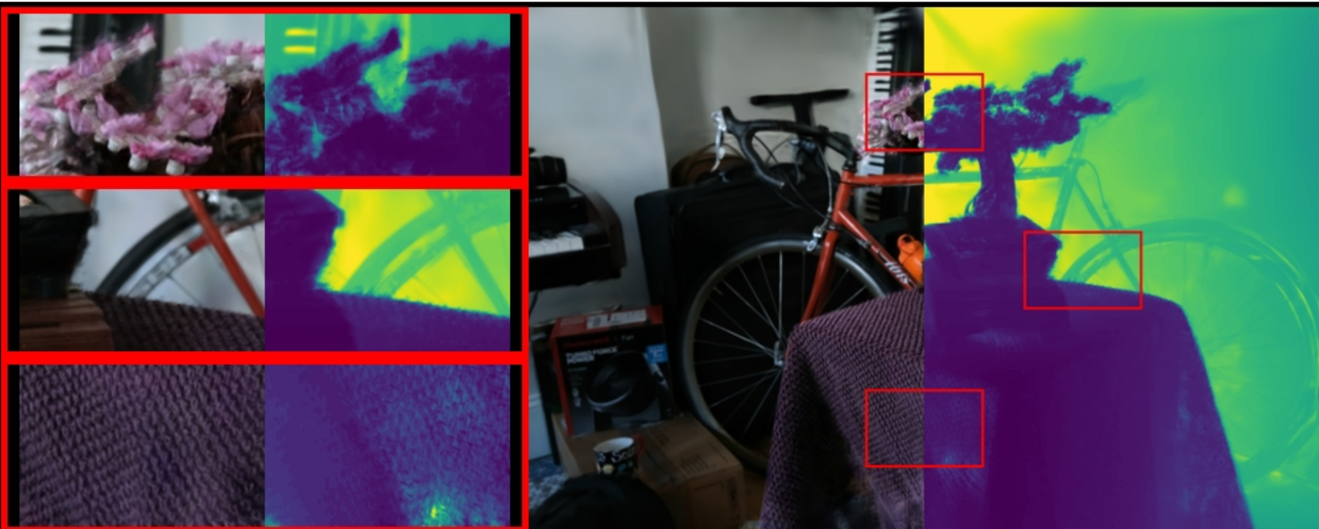
bonsai: VGGT | depth_lambda=10.0 PSNR: 18.49 | LPIPS: 0.3481 | SSIM: 0.5806
