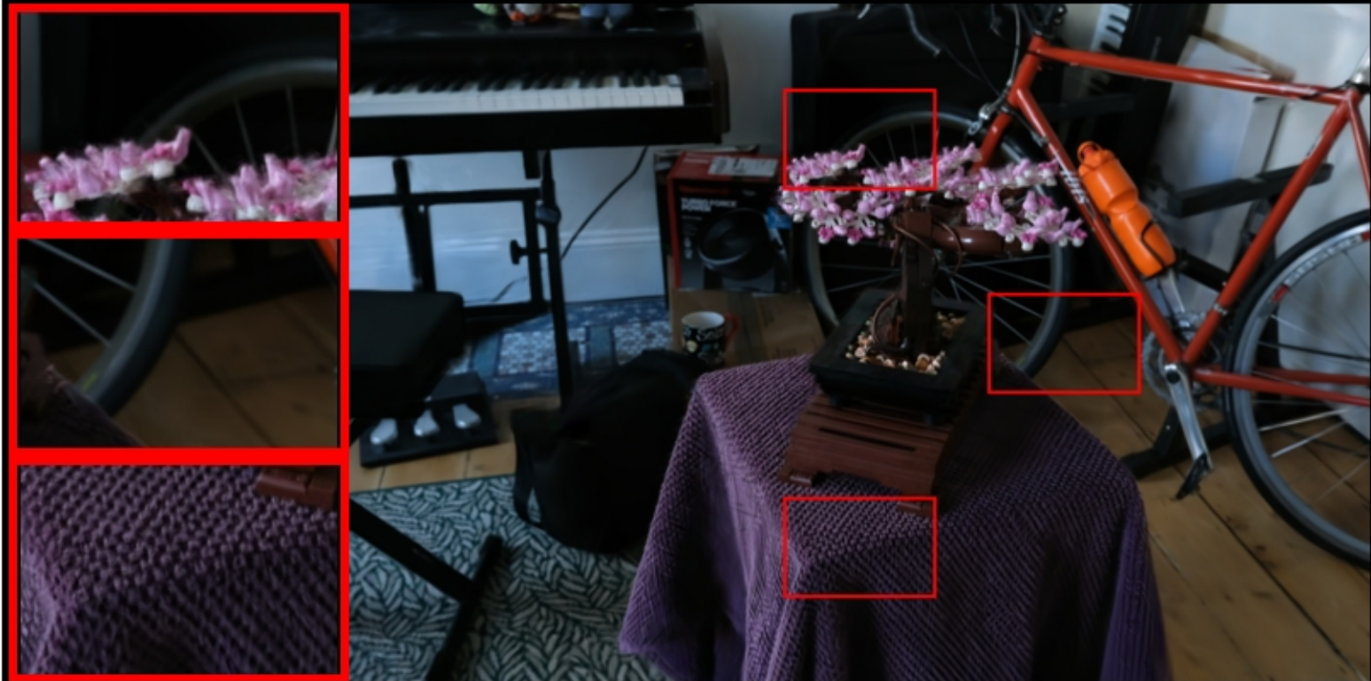
bonsai: VGGT | Random Init | Use BA PSNR: 19.73 | LPIPS: 0.3229 | SSIM: 0.6167
