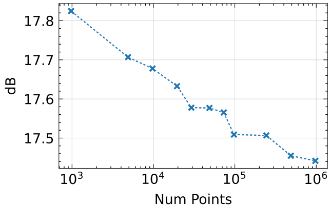
PSNR \uparrow
