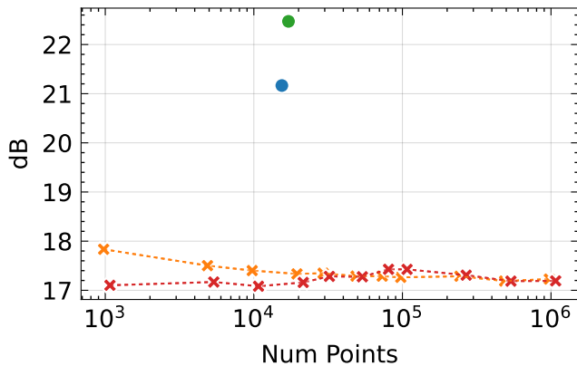
PSNR \uparrow
