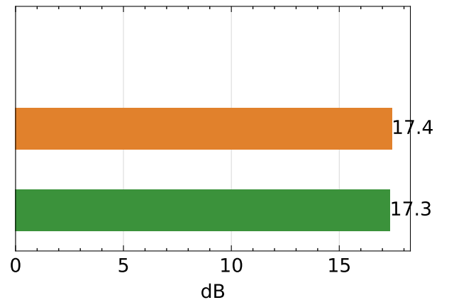
PSNR ↑
