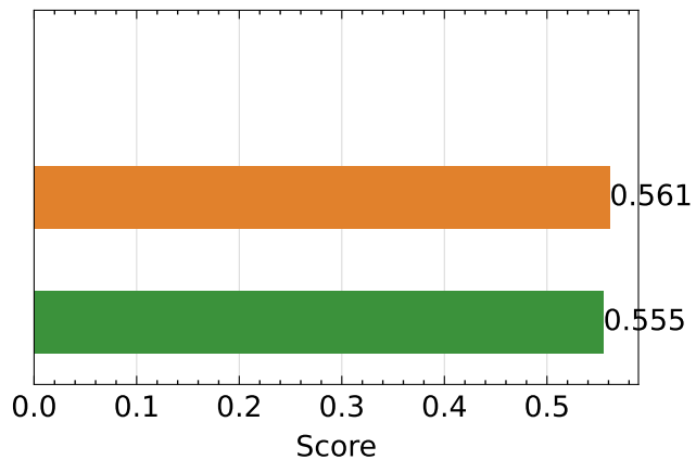
SSIM ↑
